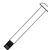
Ⓑ FAN SCREW LG600 240 X 8 PCS LG600 360 X 12 PCS
